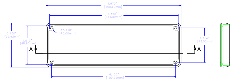
PLASTIC BEZEL
