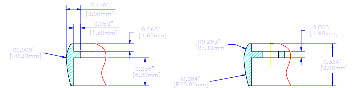
SECTION A-A SCALE 2:1
