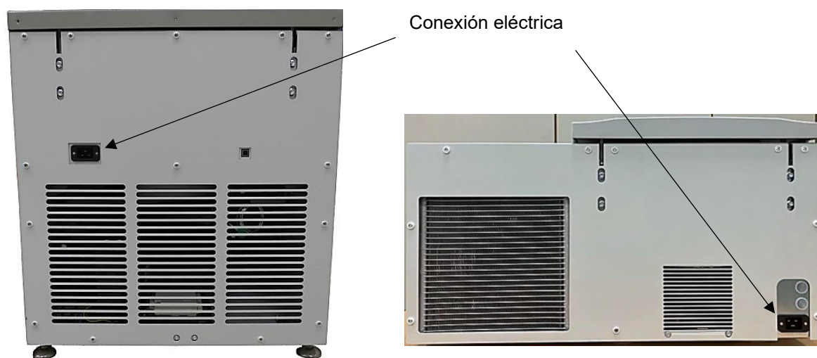
Figura 13 - Conexión eléctrica
