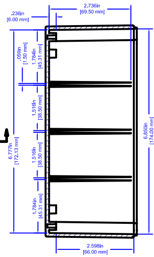
SECTION G-G SCALE 1 : 1
