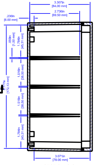
SECTION G-G SCALE 1 : 1
