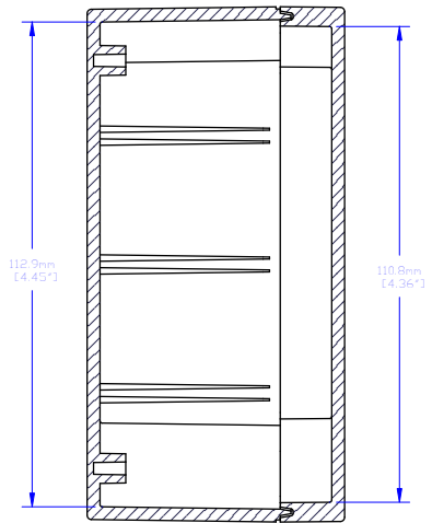
SECTION G-G SCALE 1 : 1
