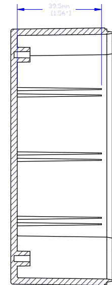
SECTION D-D SCALE 1 : 1
